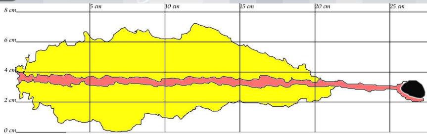
A gömblövedék útja a ballisztikai zselatinban - rövid út, gyors energialeadás
